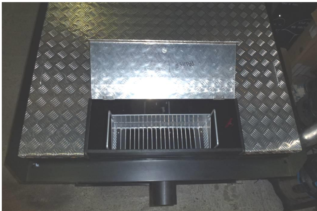
Trappe d'accès au panier dégrilleur pour une chasse de 1500 x 1130, Volume maximum 900 litres.
